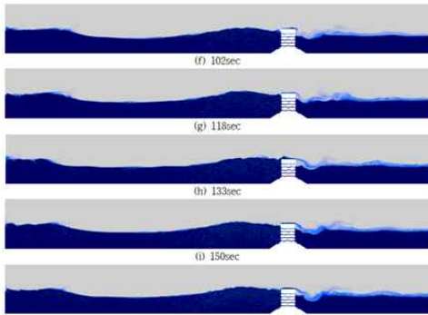
Fig. 2-11 해수소통형 블록식 케이슨
